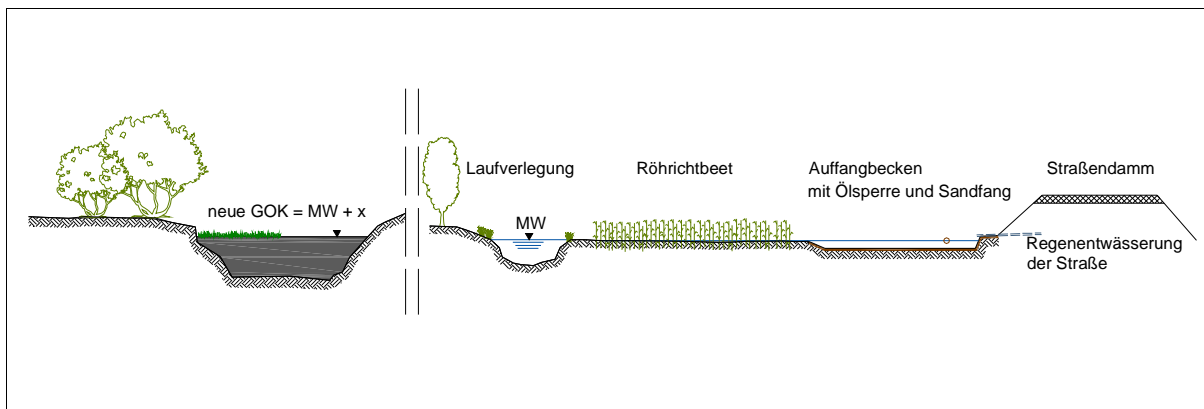
Abbildung 7-3: Prinzipskizze (Variante 1) DE588_41_P02_M03: Querprofil darstellung zur Maßnahme von Altarmanschlüssen - Regenwasserüberleitungen (Quelle: eigene Darstellung)
