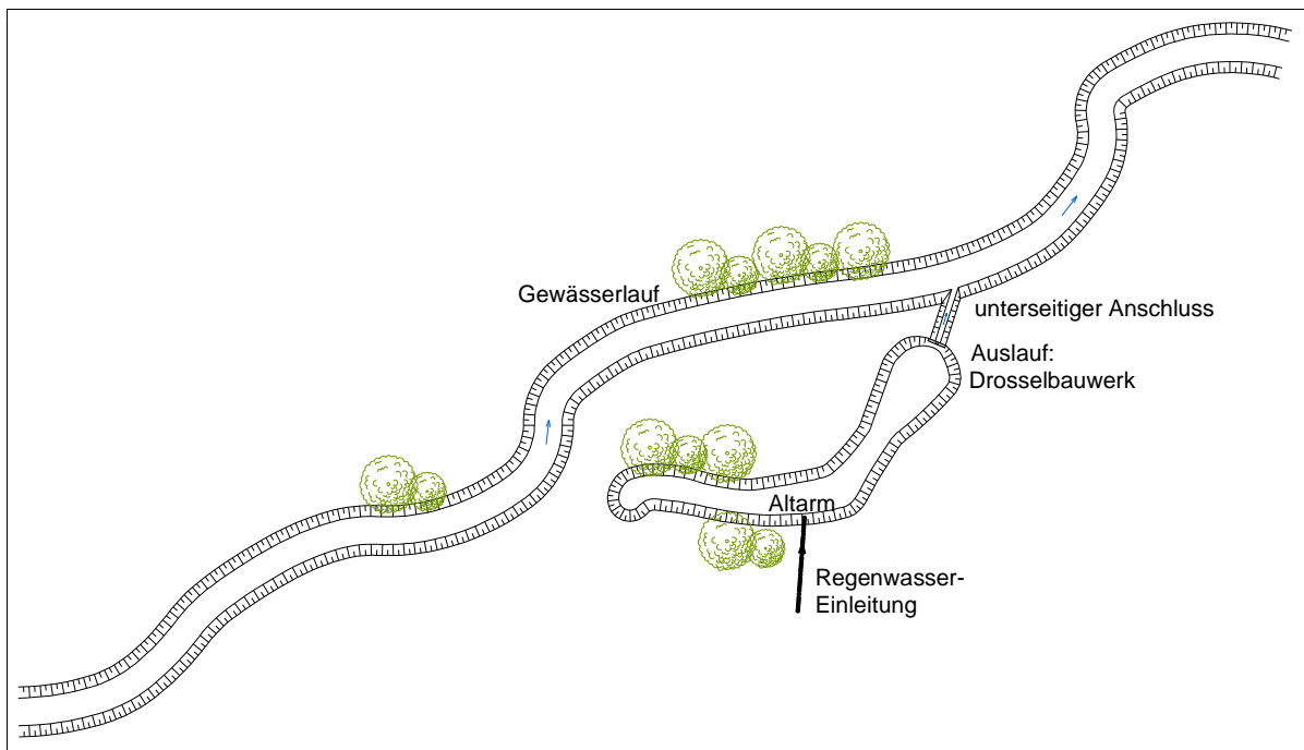
Abbildung 7-5: Prinzipskizze (Variante 2) –DE588_41_P02_M16: Darstellung der Altarmgestaltung als Regenrückhaltebecken (Quelle: eigene Darstellung)
