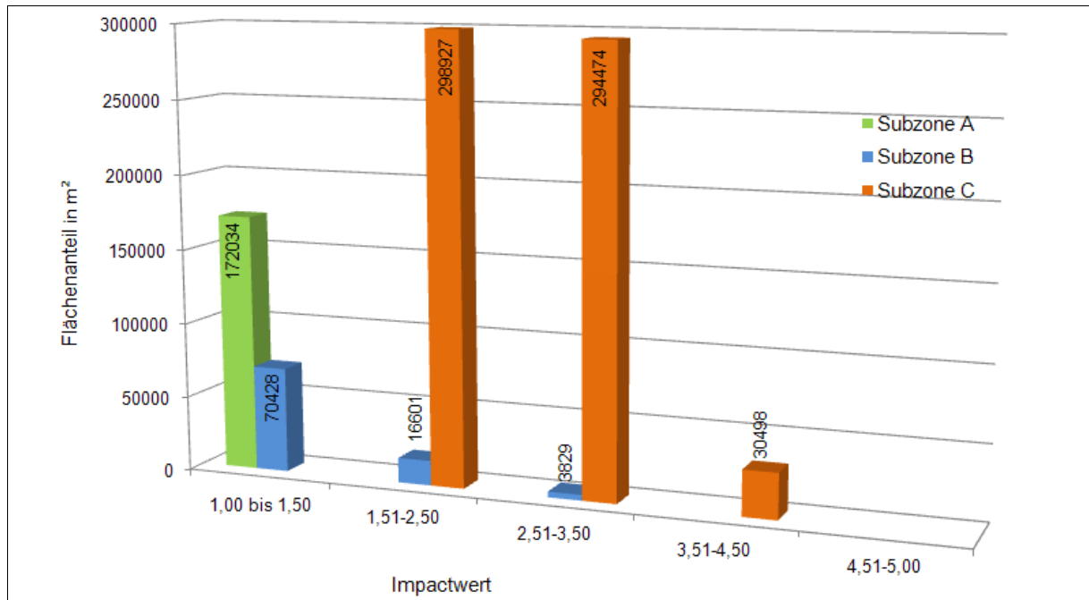
Abbildung 3-20: Diagramm über die Verteilung entsprechend den Impactwerten (Güteklassen) der Seeuferbewertung bezogen auf die festgelegten Subzonenflächen des Siethener Sees
