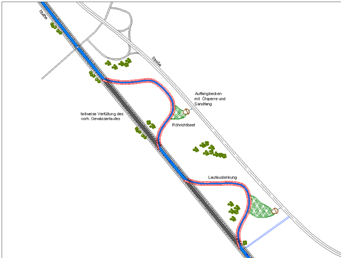
Abbildung 7-4: Prinzipskizze (Variante 1) DE588_41_P02_M03: Darstellung zur Maßnahme von Altarmanschlüssen – Regenwasserüberleitungen (Quelle: eigene Darstellung)
