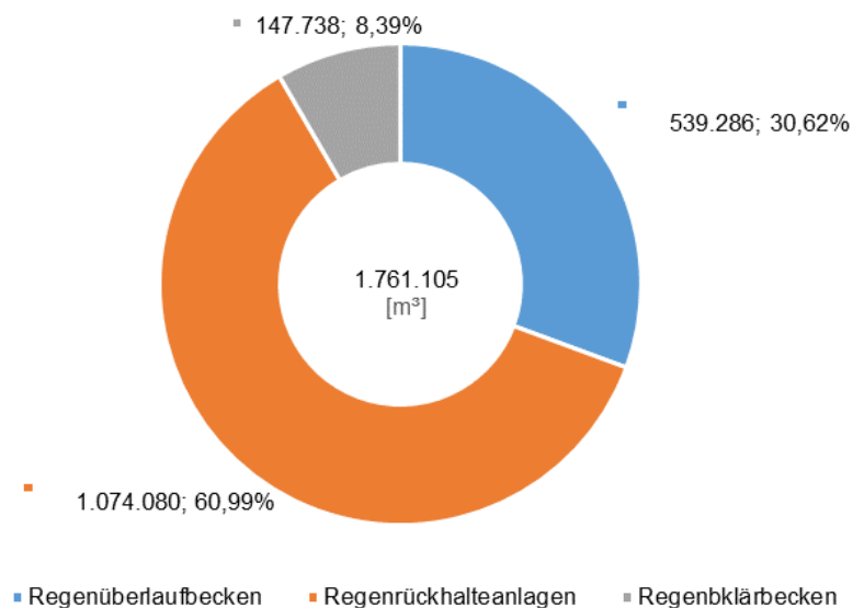
Abbildung 3-149: Speichervolumen der Regentlastungsbauwerke FGE Maas (Stand 2016)
