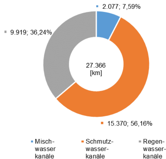
Abbildung 3-128: Länge der öffentlichen Kanalisation FGE Ems (Stand 2016)
