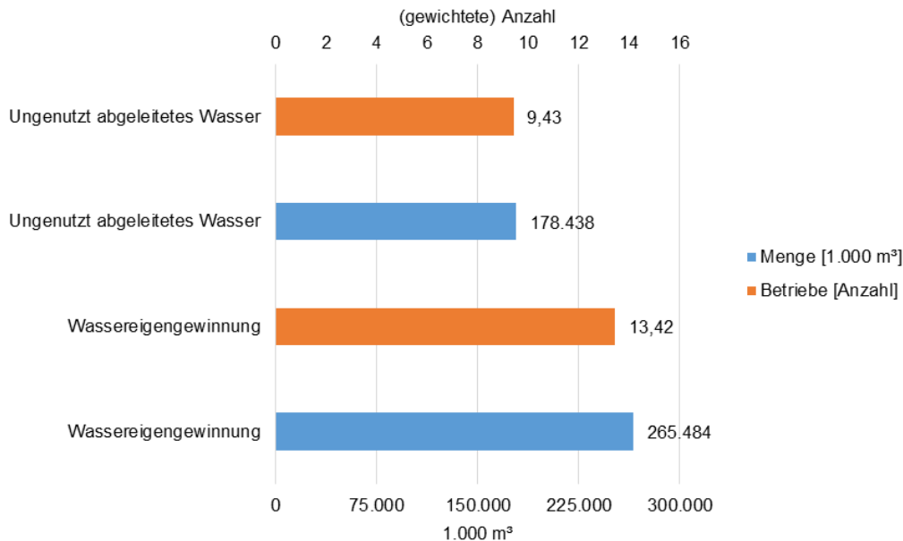
Abbildung 3-181: Kohlebergbau, Gewinnung von Erdöl und Erdgas, Erzbergbau: Wassergewinnung sowie ungenutzt abgeleitetes Wasser in Betrieben FGE Rhein (Stand 2016) 13
