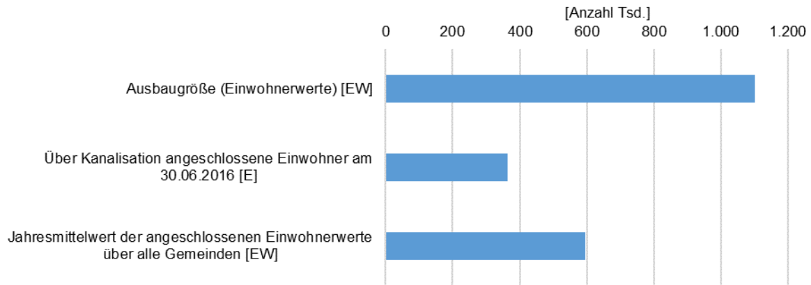
Abbildung 3-89: Ausbaugröße, angeschlossene Einwohner und angeschlossene Einwohnerwerte FGE Eider (Stand 2016)
