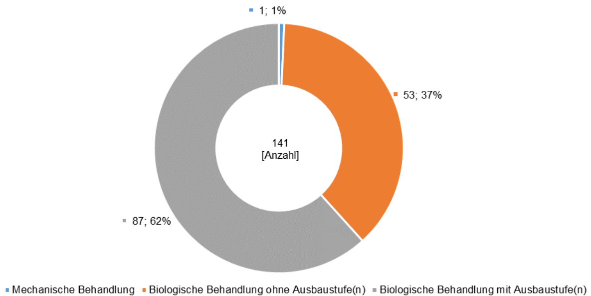
Abbildung 3-82: Anzahl der Kläranlagen nach Art des Reinigungsverfahrens FGE Oder (Stand 2016)
