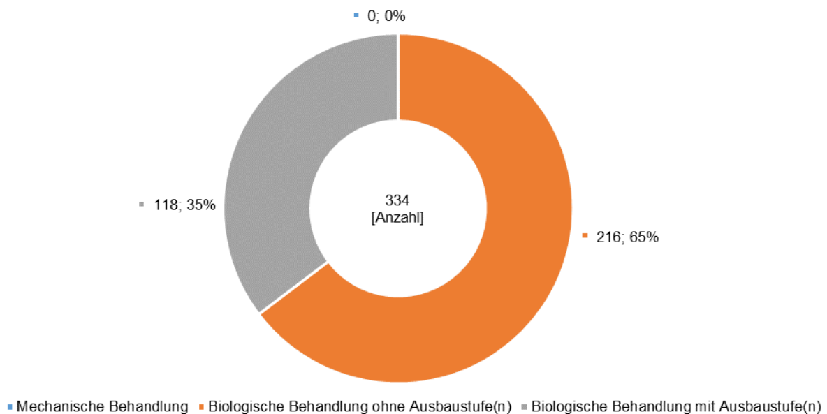
Abbildung 3-90: Anzahl der Kläranlagen nach Art des Reinigungsverfahrens FGE Schlei/Trave (Stand 2016)
