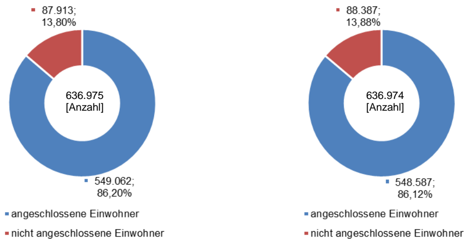
Abbildung 3-116: Anschlussverhältnisse der öffentlichen Kanalisation (links) und Zentralen Kläranlagen (rechts) FGE Oder (Stand 2016)
