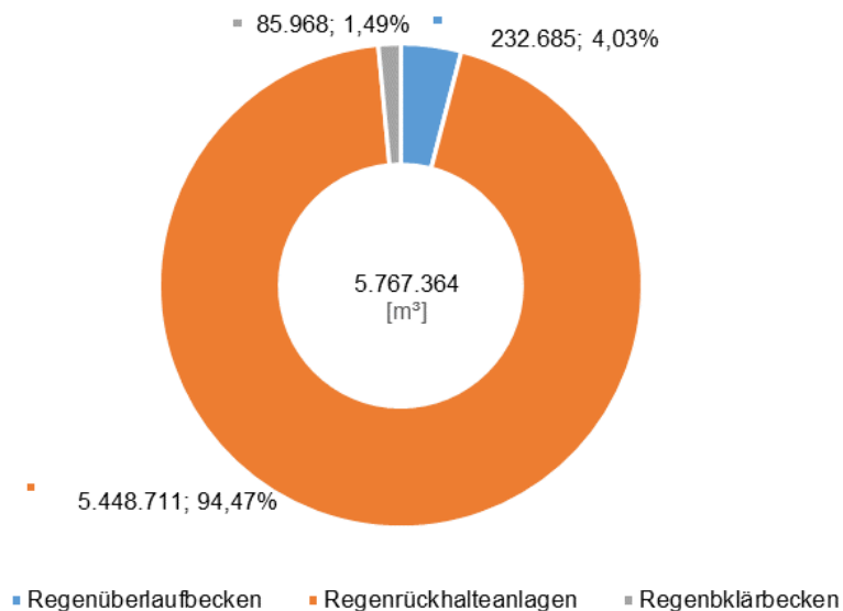
Abbildung 3-141: Speichervolumen der Regentlastungsbauwerke FGE Ems (Stand 2016)
