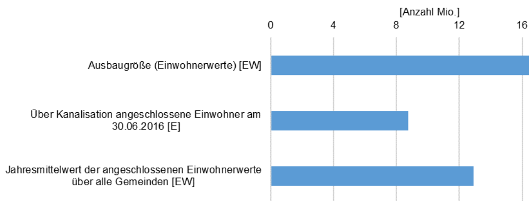
Abbildung 3-78: Ausbaugröße, angeschlossene Einwohner und angeschlossene Einwohnerwerte FGE Weser (Stand 2016)
