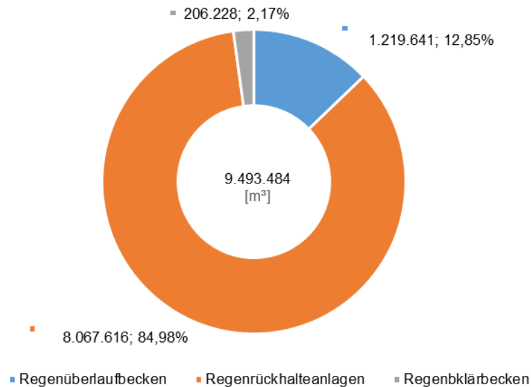
Abbildung 3-143: Speichervolumen der Regentlastungsbauwerke FGE Weser (Stand 2016)
