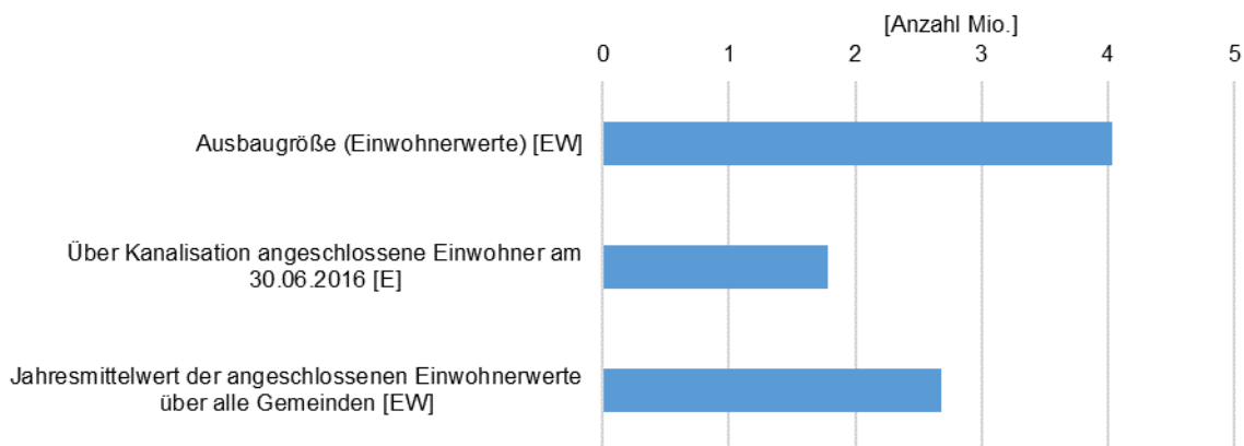
Abbildung 3-86: Ausbaugröße, angeschlossene Einwohner und angeschlossene Einwohnerwerte FGE Maas (Stand 2016)
