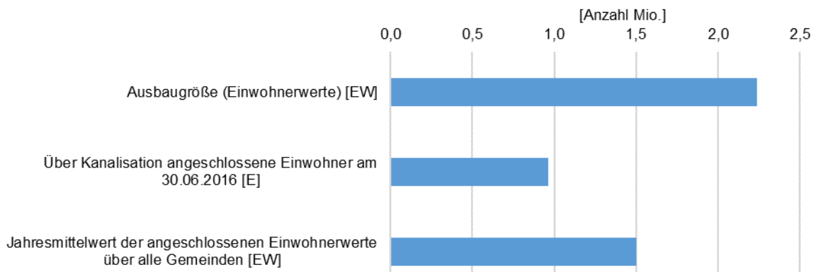
Abbildung 3-95: Ausbaugröße, angeschlossene Einwohner und angeschlossene Einwohnerwerte FGE Warnow/Peene (Stand 2016)
