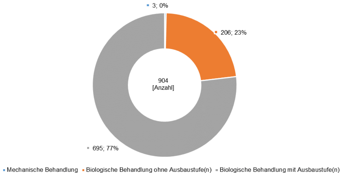
Abbildung 3-76: Anzahl der Kläranlagen nach Art des Reinigungsverfahrens FGE Weser (Stand 2016)
