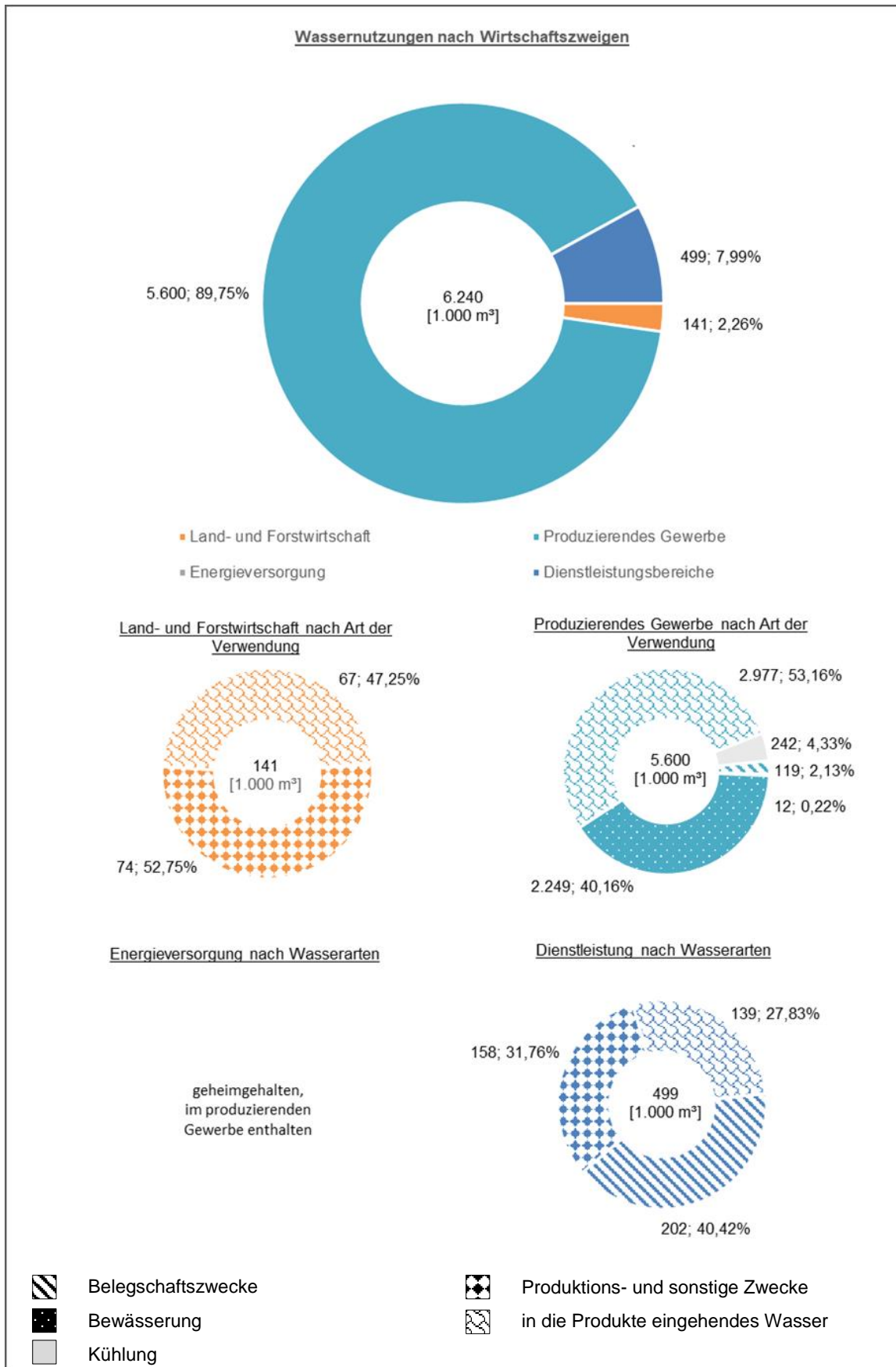
Abbildung 3-177: Wassereinsatz in Betrieben nach Art der Verwendung und Wirtschaftszweigen und Energieversorgung und Dienstleistung nach Art der Verwendung FGE Eider (Stand 2016)
