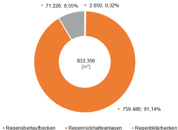
Abbildung 3-151: Speichervolumen der Regentlastungsbauwerke FGE Eider (Stand 2016)
