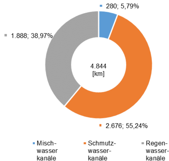
Abbildung 3-133: Länge der öffentlichen Kanalisation FGE Eider (Stand 2016)
