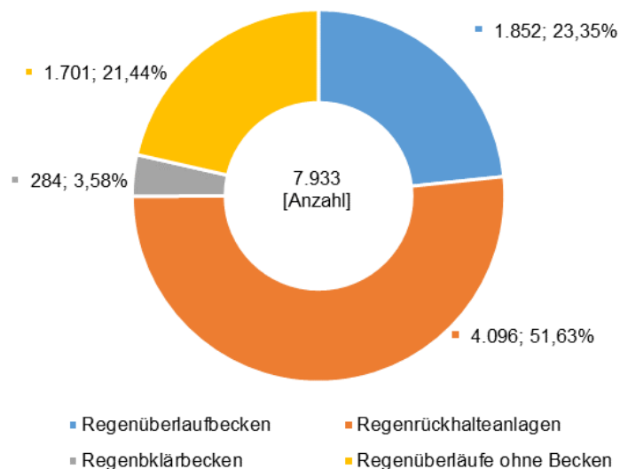
Abbildung 3-142: Anzahl der Regentlastungsbauwerke FGE Weser (Stand 2016)
