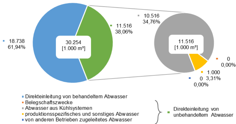
Abbildung 3-204: Verbleib des Abwassers des produzierenden Gewerbes FGE Oder nach seiner Herkunft (Stand 2016)
