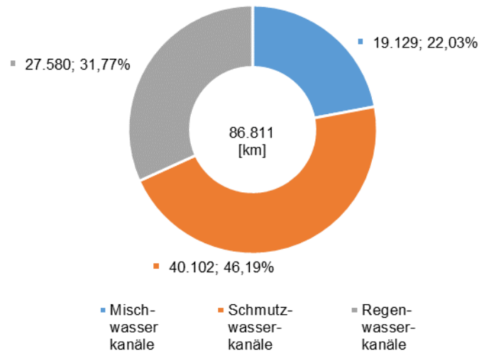
Abbildung 3-129: Länge der öffentlichen Kanalisation FGE Weser (Stand 2016)
