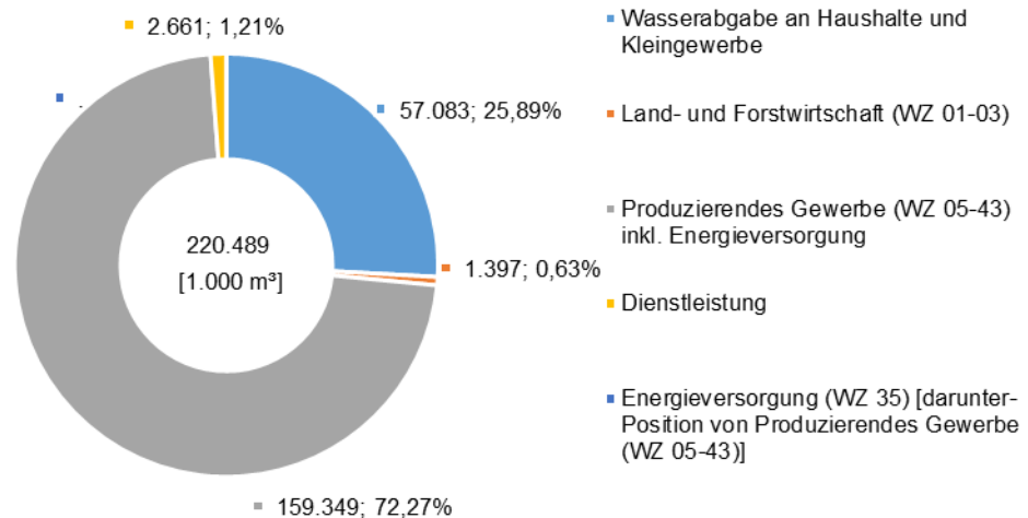
Abbildung 3-50: Wassereinsatz nach Bereichen in der FGE Schlei/Trave (Stand 2016)
