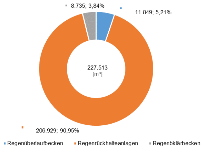
Abbildung 3-147: Speichervolumen der Regentlastungsbauwerke FGE Oder (Stand 2016)
