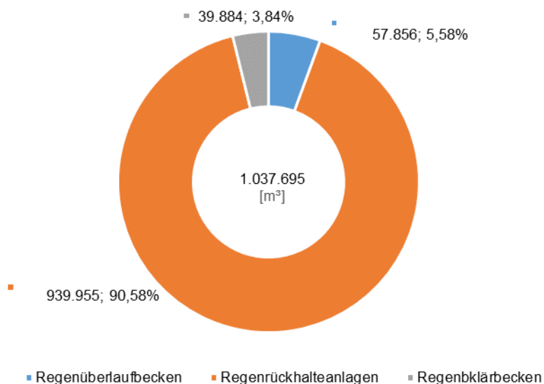
Abbildung 3-155: Speichervolumen der Regenentlastungsbauwerke FGE Warnow/Peene (Stand 2016)
