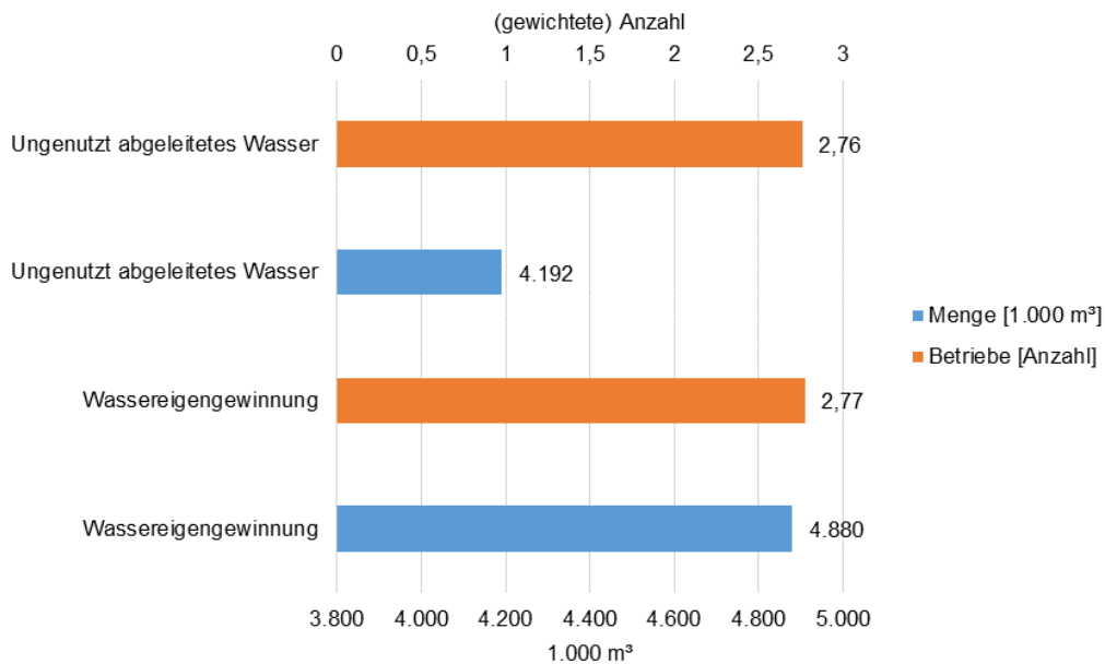
Abbildung 3-185: Kohlebergbau, Gewinnung von Erdöl und Erdgas, Erzbergbau: Wassergewinnung sowie ungenutzt abgeleitetes Wasser in Betrieben FGE Weser (Stand 2016) 15
