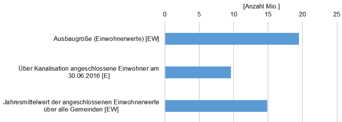
Abbildung 3-69: Ausbaugröße, angeschlossene Einwohner und angeschlossene Einwohnerwerte FGE Donau (Stand 2016)
