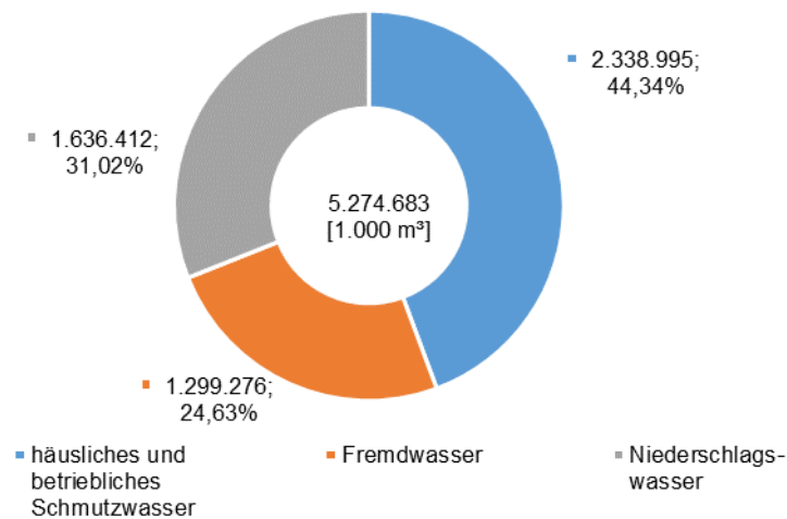
Abbildung 3-97: Abwassermengen nach Herkunft FGE Rhein (Stand 2016)
