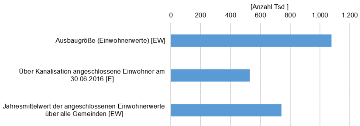
Abbildung 3-84: Ausbaugröße, angeschlossene Einwohner und angeschlossene Einwohnerwerte FGE Oder (Stand 2016)
