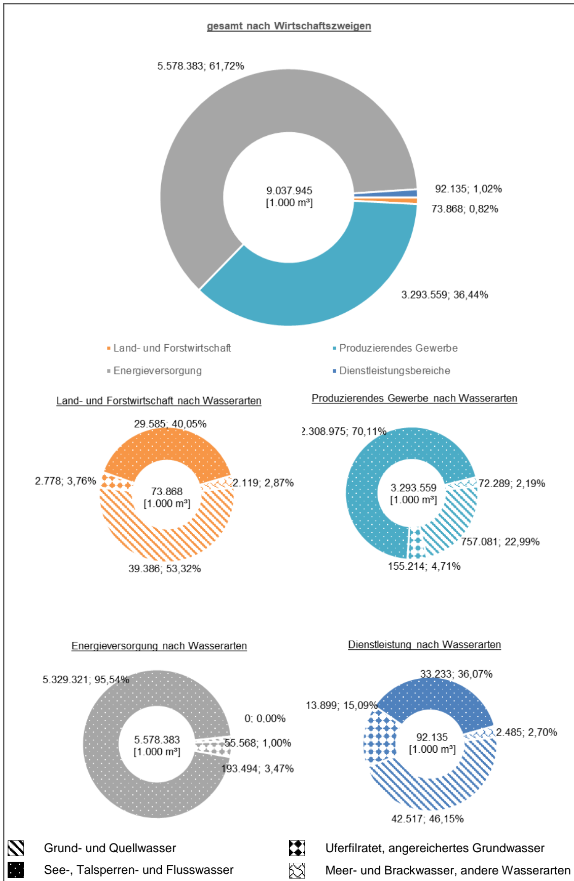
Abbildung 3-161: Wassereigengewinnung in Betrieben nach Wirtschaftszweigen und Wasserarten FGE Rhein (Stand 2016)
