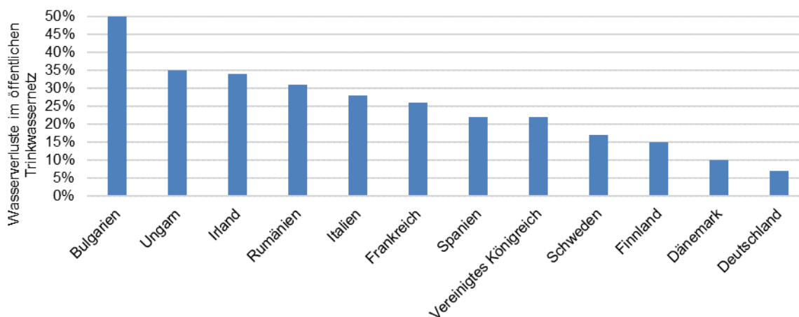
Abbildung 4-6: Wasserverluste im öffentlichen Trinkwassernetz als wichtigster Indikator für Qualität des Netzes und Versorgungssicherheit im internationalen Vergleich 27 (Wasserverluste in ausgewählten europäischen Ländern (in Prozent vom Bruttowasseraufkommen), 2008)
