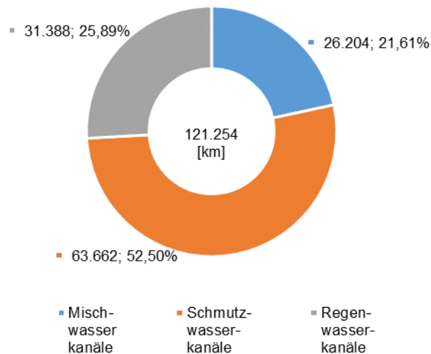
Abbildung 3-130: Länge der öffentlichen Kanalisation FGE Elbe (Stand 2016)
