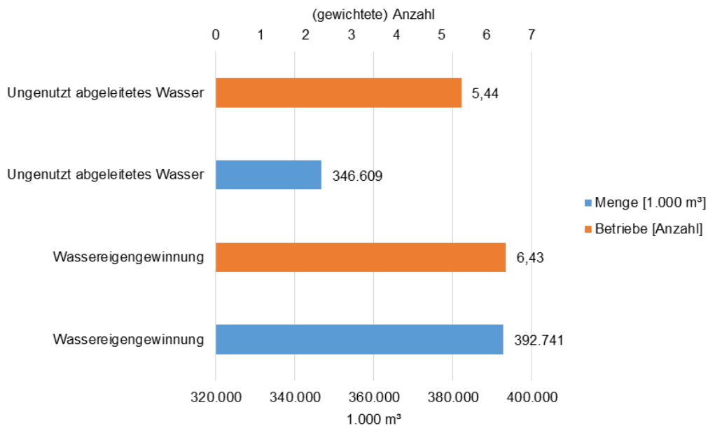
Abbildung 3-187: Kohlebergbau, Gewinnung von Erdöl und Erdgas, Erzbergbau: Wassergewinnung sowie ungenutzt abgeleitetes Wasser in Betrieben FGE Elbe (Stand 2016) 16
