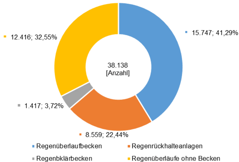
Abbildung 3-138: Anzahl der Regentlastungsbauwerke FGE Rhein (Stand 2016)
