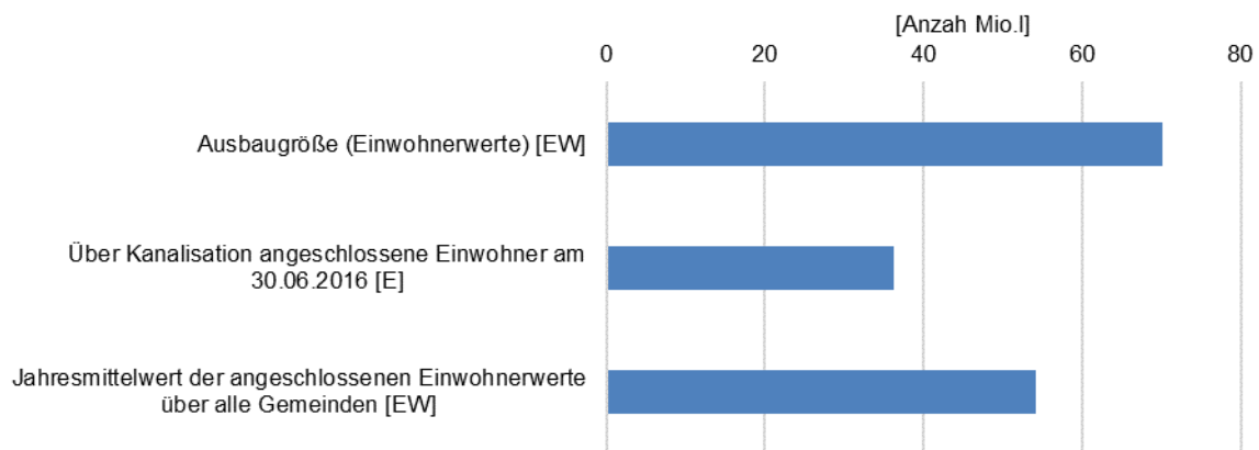
Abbildung 3-72: Ausbaugröße, angeschlossene Einwohner und angeschlossene Einwohnerwerte FGE Rhein (Stand 2016)
