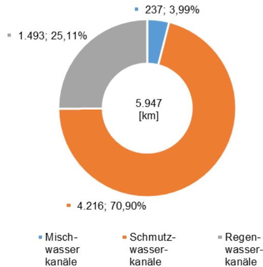
Abbildung 3-131: Länge der öffentlichen Kanalisation FGE Oder (Stand 2016)
