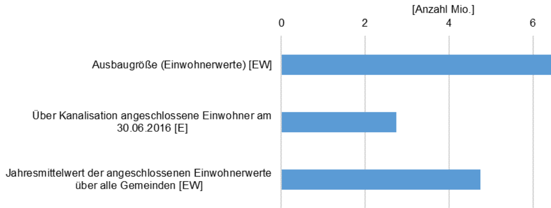
Abbildung 3-75: Ausbaugröße, angeschlossene Einwohner und angeschlossene Einwohnerwerte FGE Ems (Stand 2016)
