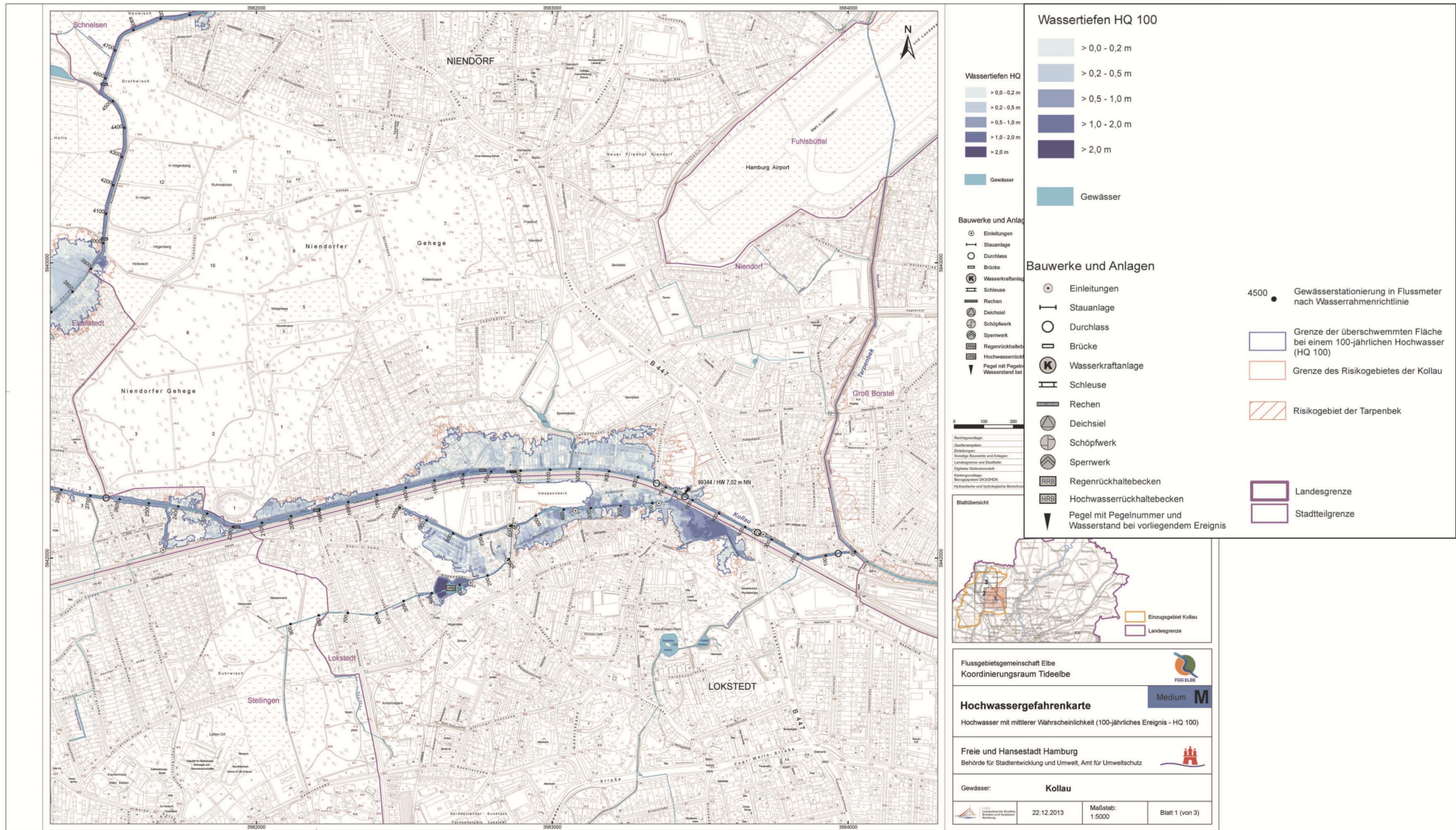
Abb. 2.3.1-5: Beispiel für eine Hochwassergefahrenkarte – Hamburg (Quelle: BUE, Hamburg)
