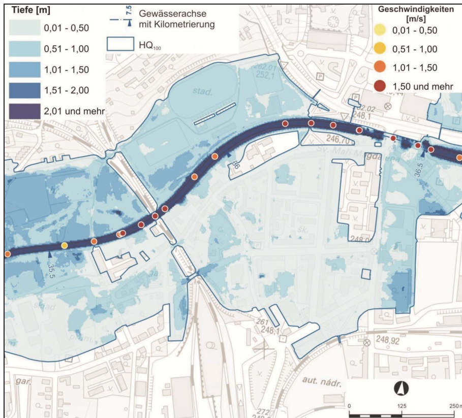
Abb. 2.3.1-2: Ausschnitt einer Karte mit den Tiefen und Geschwindigkeiten für ein Hochwasserszenario mit einem Wiederkehrintervall von 100 Jahren ( HQ_{100} ) – Ergebnis des eindimensionalen Modells (Quelle: Povodí Ohře, s. p.)
