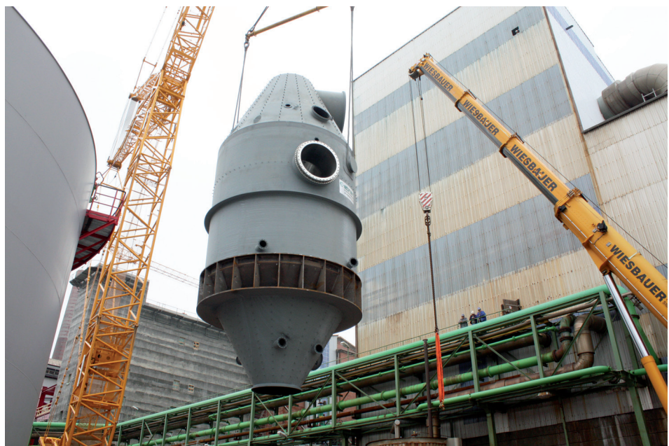
Einbau einer Eindampfanlage am Standort Wintershall zur Einbindung von Salzabwässern aus Unterbreizbach
