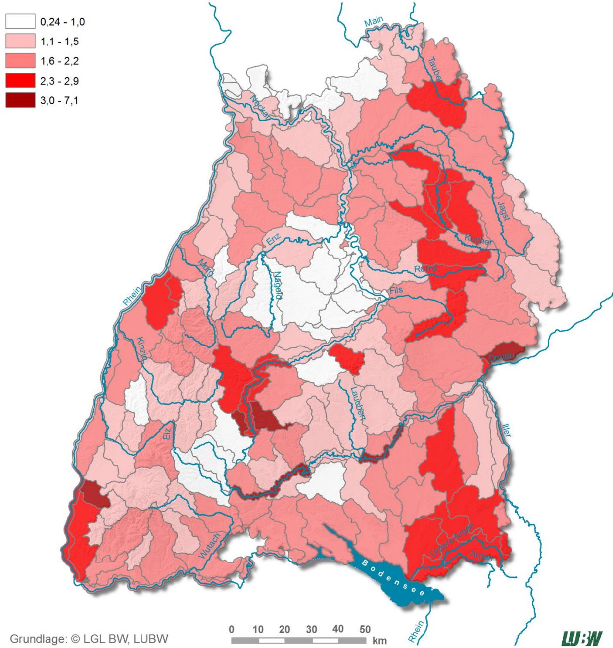
Abbildung 12: Flächenspezifische Stickstoff-Einträge über diffuse Quellen auf Wasserkörperenebene [t/(km 2 ·a)]
