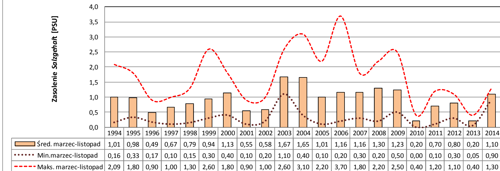
Zasolenie (marzec-listopad) - Stanowisko C - warstwa powierzchniowa, Zalew Wielki, Salzgehalt (März bis November) - Station C - Oberfläche, Großes Haff, 1994-2014
