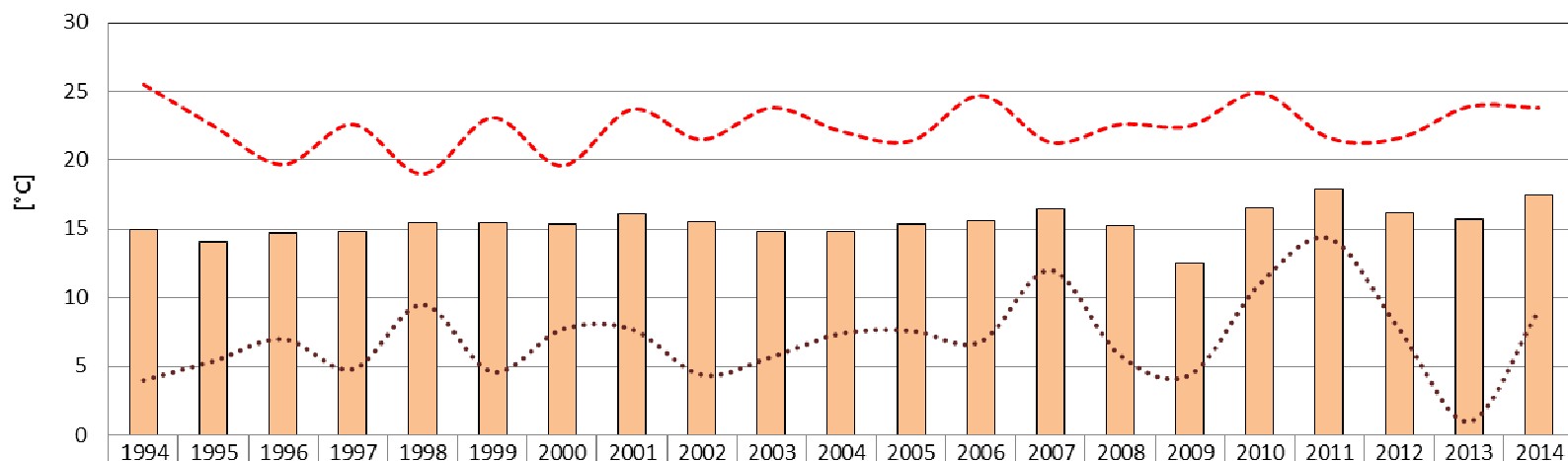
Temperatura wody (warstwa powierzchniowa, średnia roczna) Stanowisko C, Zalew Wielki, Wassertemperatur (Oberfläche, Jahresmittel) Station C, Großes Haff, 1994 - 2014
