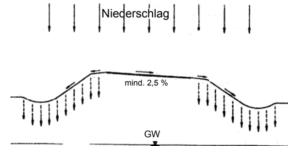
b 2 ) Versickerung in Mulden
