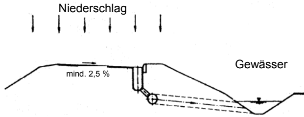
a 1 ) direkte Einleitung in Gewässer
