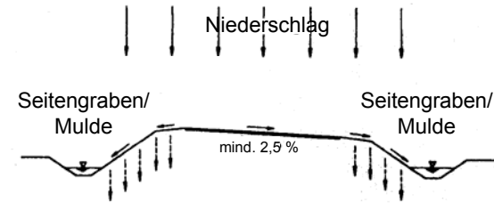
b 1 ) Einleitung in Mulden/Seitengraben
