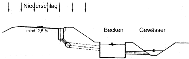
a 2 ) Einleitung über Becken in Gewässer
